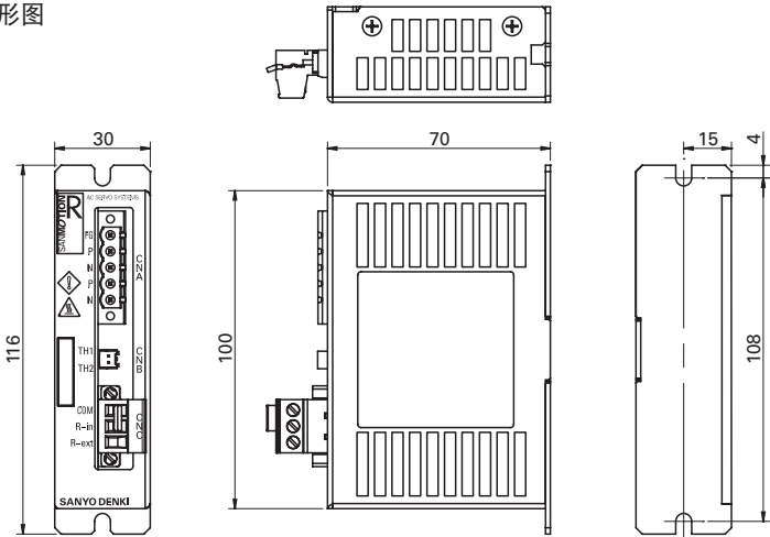
外形图
