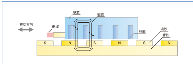
电机横截面（侧视图）
