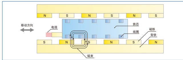
电机横截面（俯视图）
